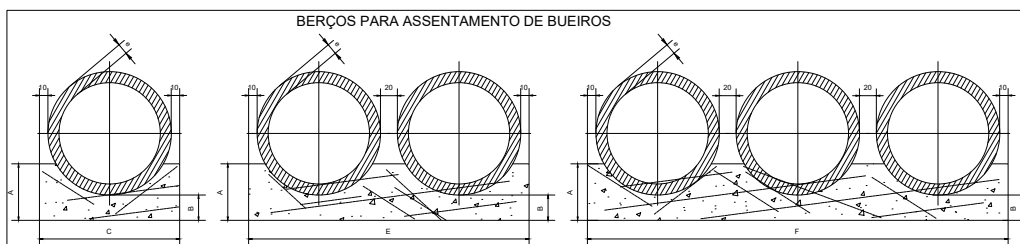
VISTA LATERAL
