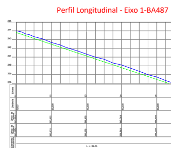
Perfil Longitudinal - Eixo 1-BA487
