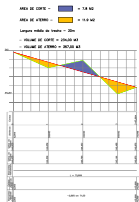
Perfil Longitudinal - Eixo 01-Mercado - Greide de Pavimento Acabado
