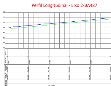
Perfil Longitudinal - Eixo 2-BA487
