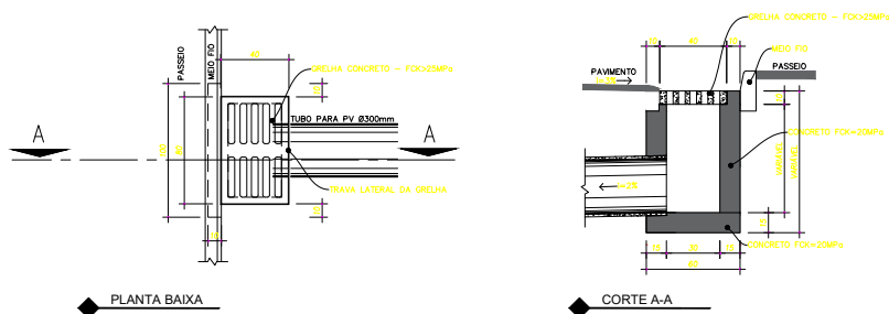
DETALHE - BOCA DE LOBO (BL)
