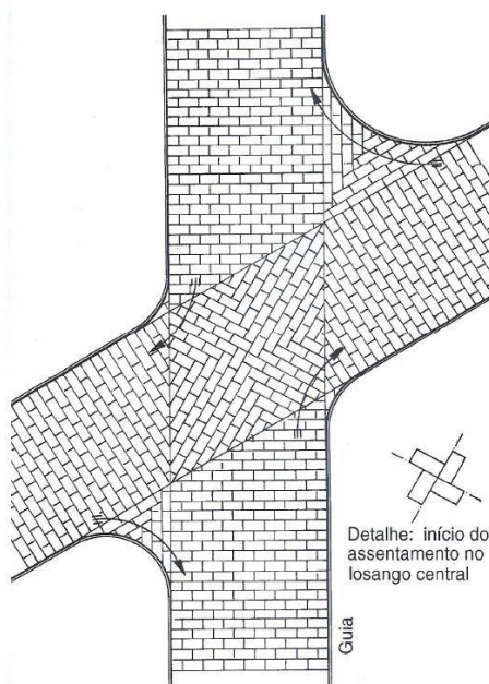
Figura 02 – Cruzamentos Esconsos
