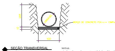
DETALHE - VALA DE ASSENTAMENTO DO TUBO
