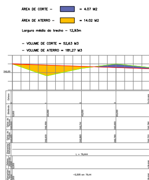
Perfil Longitudinal - Eixo 02-Mercado - Greide de Pavimento Acabado
