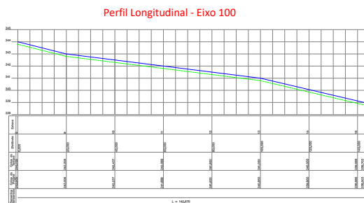
Perfil Longitudinal - Eixo 100
