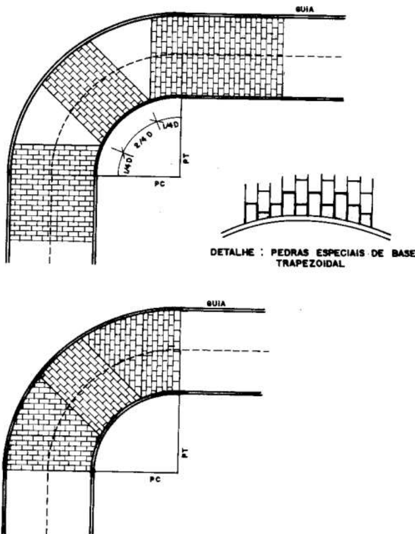
Ilustração Nº 3 Assentamento de Calçamento - Trecho em Curva de Pequeno Raio .
