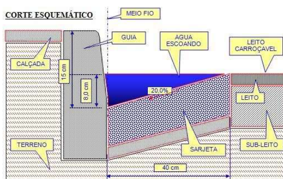
Figura 01 – Corte esquemático da pavimentação
