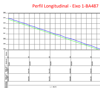
Perfil Longitudinal - Eixo 1-BA487
