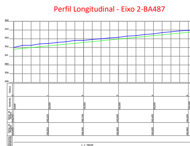
Perfil Longitudinal - Eixo 2-BA487
