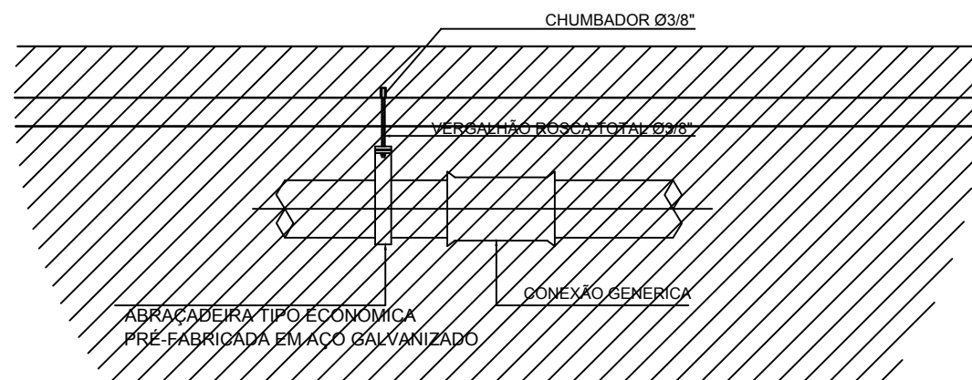
DET. LATERAL DE FIXAÇÃO DE TUBULAÇÃO NA PONTE SEM ESCALA
