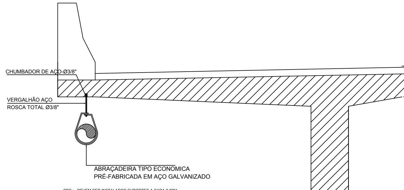
DET. DE FIXAÇÃO DE TUBULAÇÃO NA PONTE SEM ESCALA
