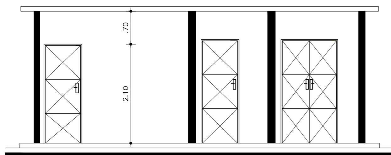
FACHADA FRONTAL
