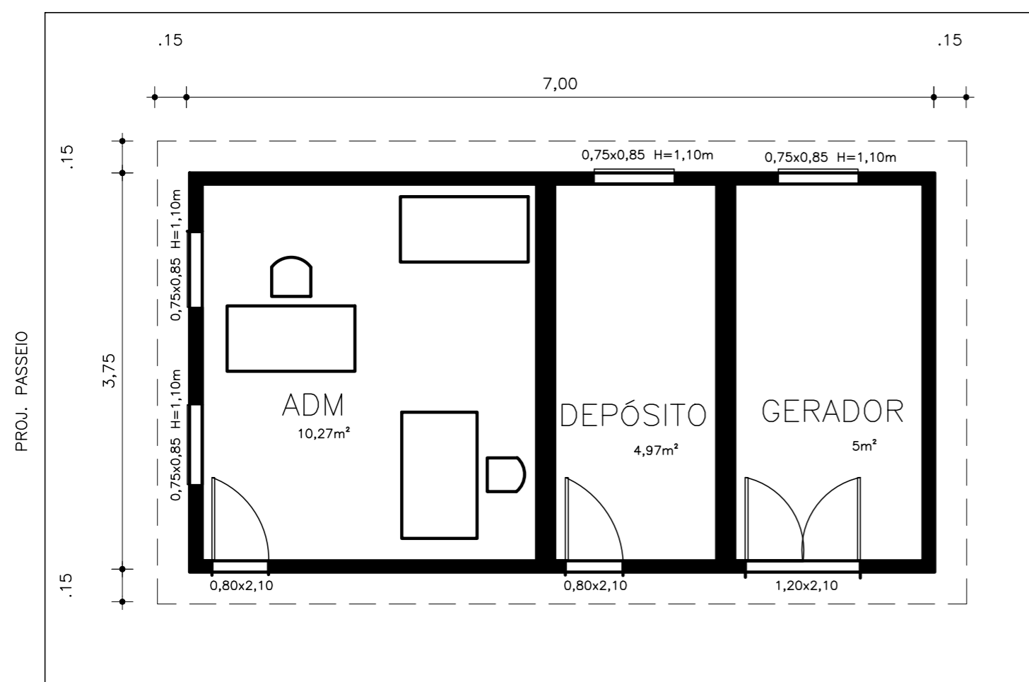
PLANTA BAIXA
