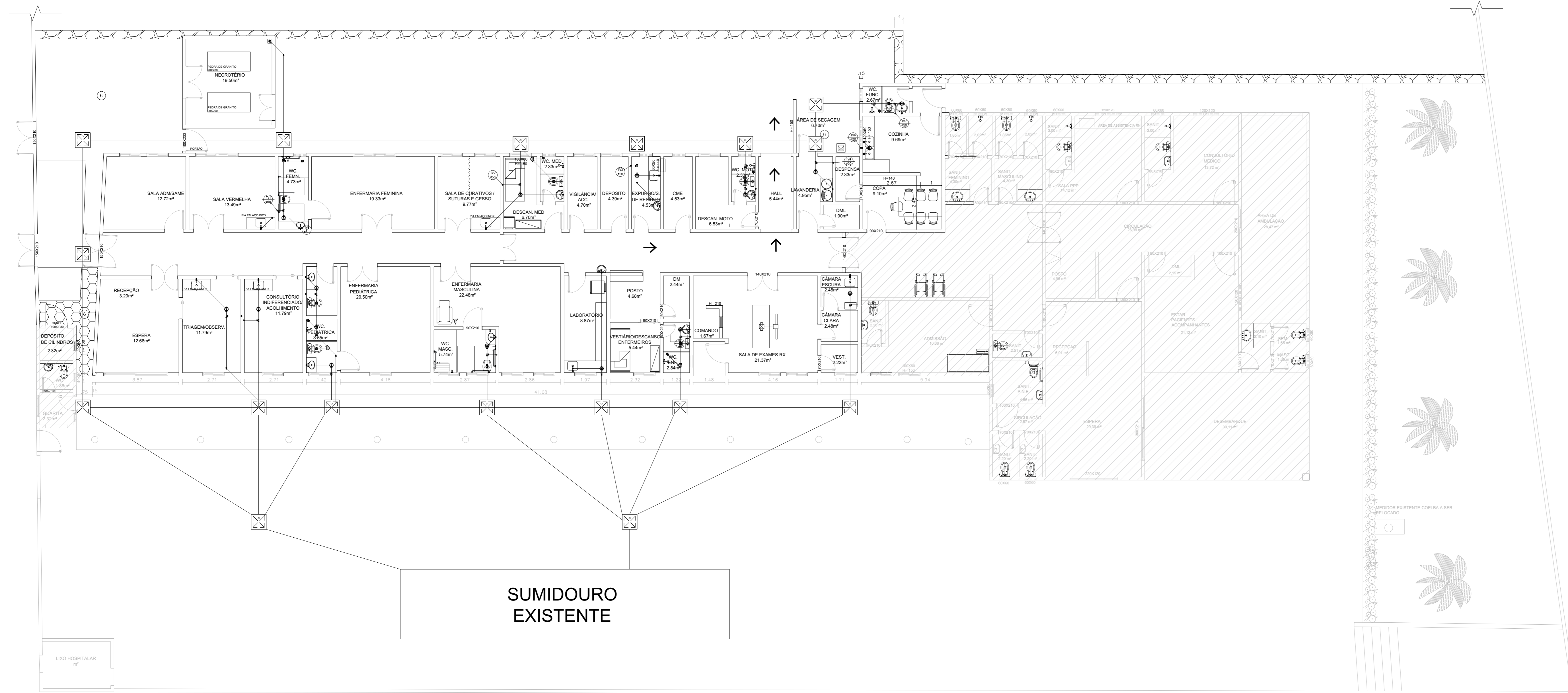
PLANTA BAIXA – GUIA DE ESGOTO 1:100
