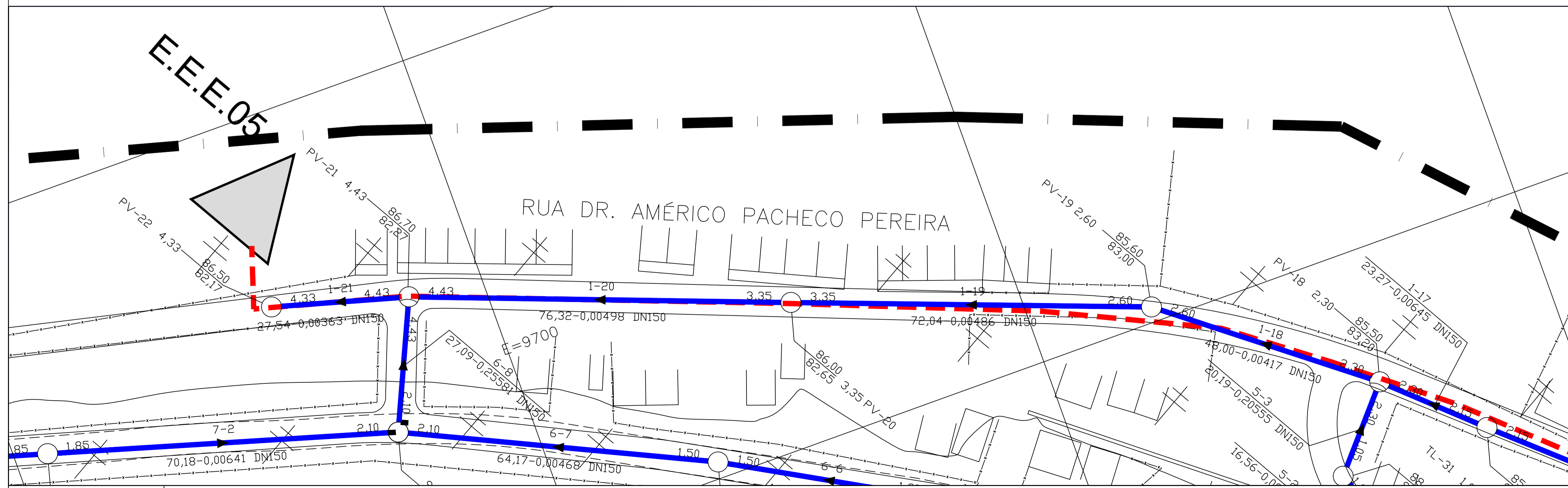
PLANTA -TRECHOS 1-19 AO 1-21 - PERFIL - PV'S 19 ao 22
