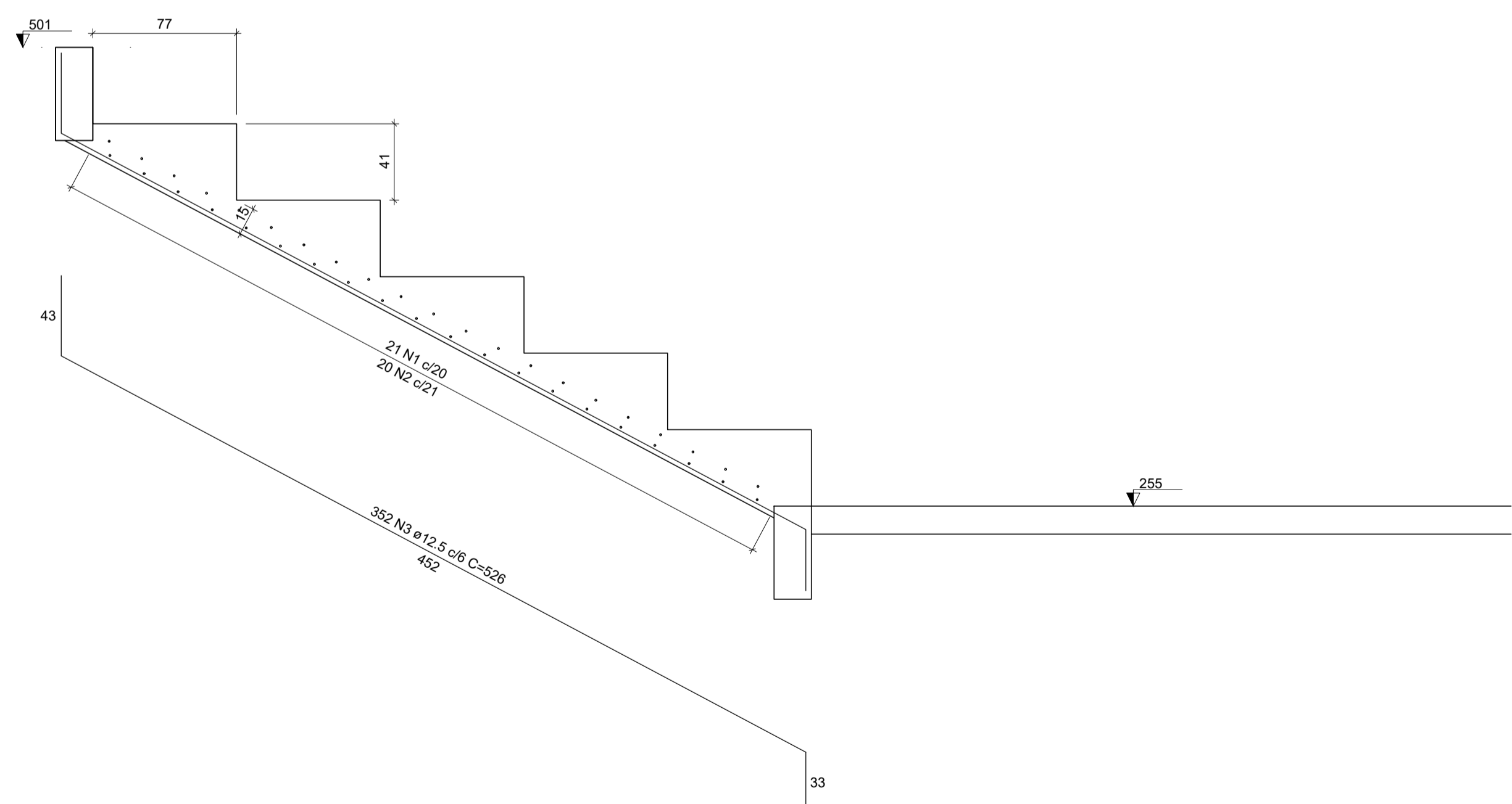
Corte A-A (LE1) ESC 1:25
