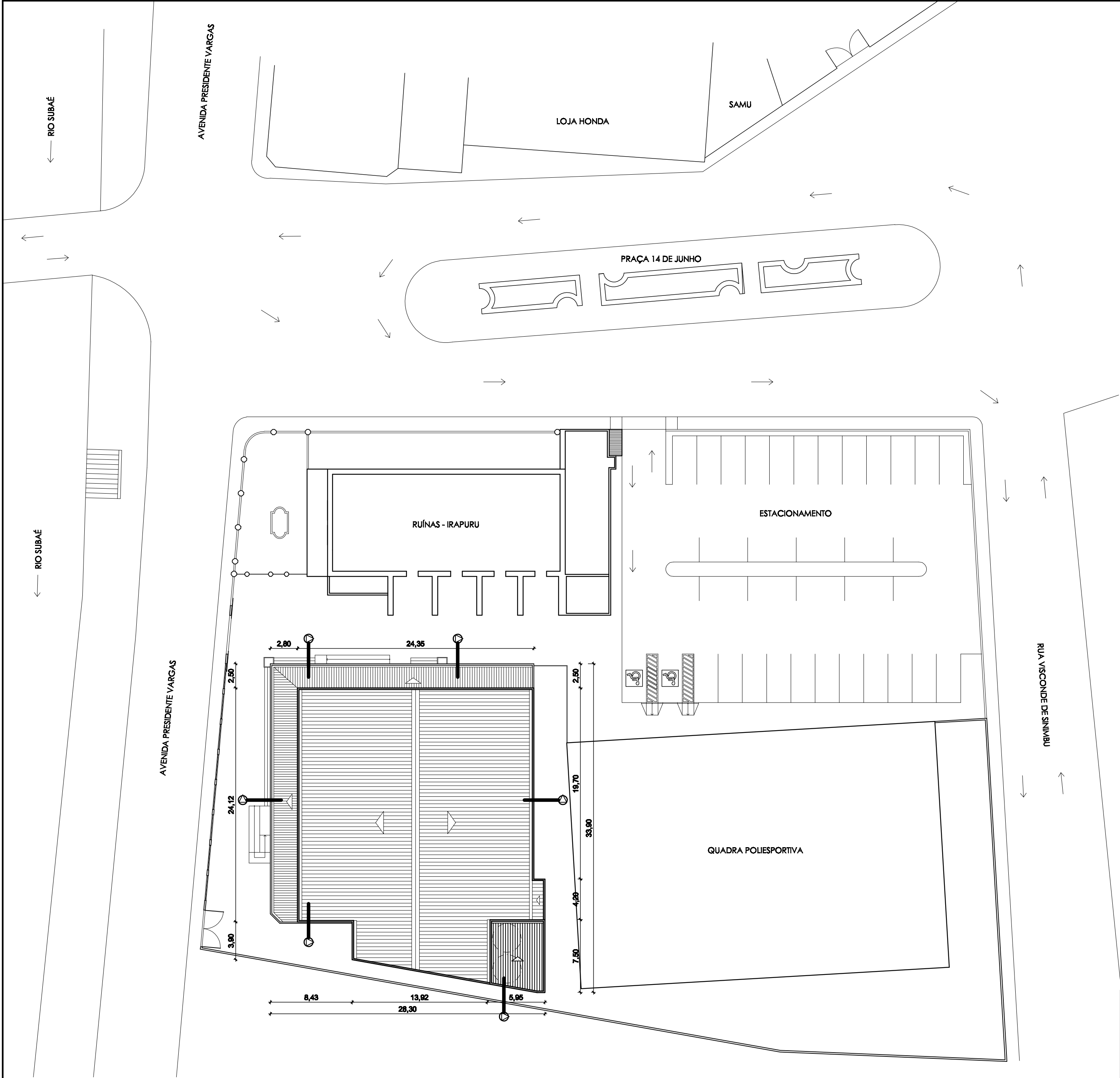
PLANTA DE SITUAÇÃO ESCALA 1/300
