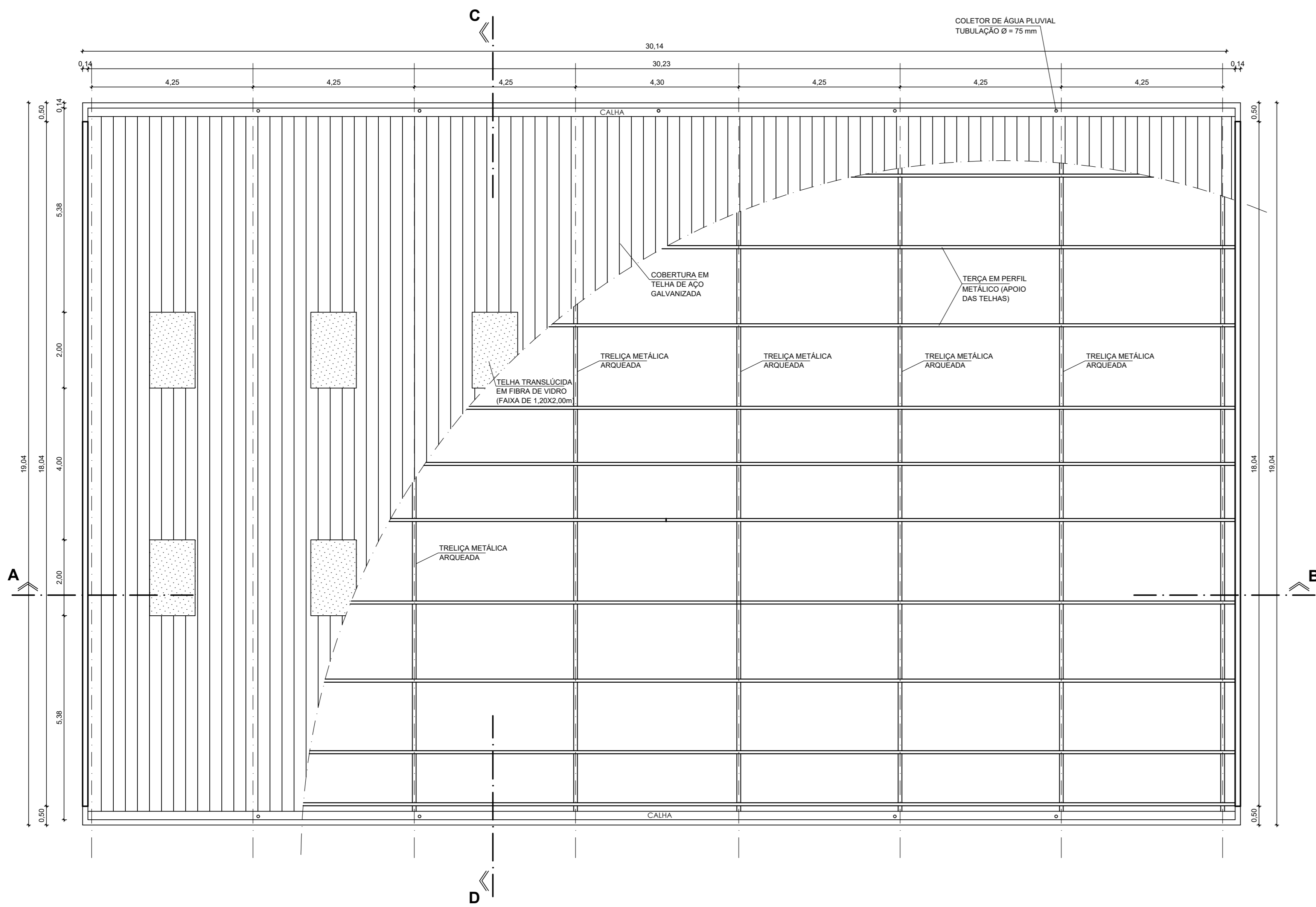
PLANTA DE COBERTURA - DIAGRAMAÇÃO DA ESTRUTURA DO TELHA DO ESCALA: 1/75
