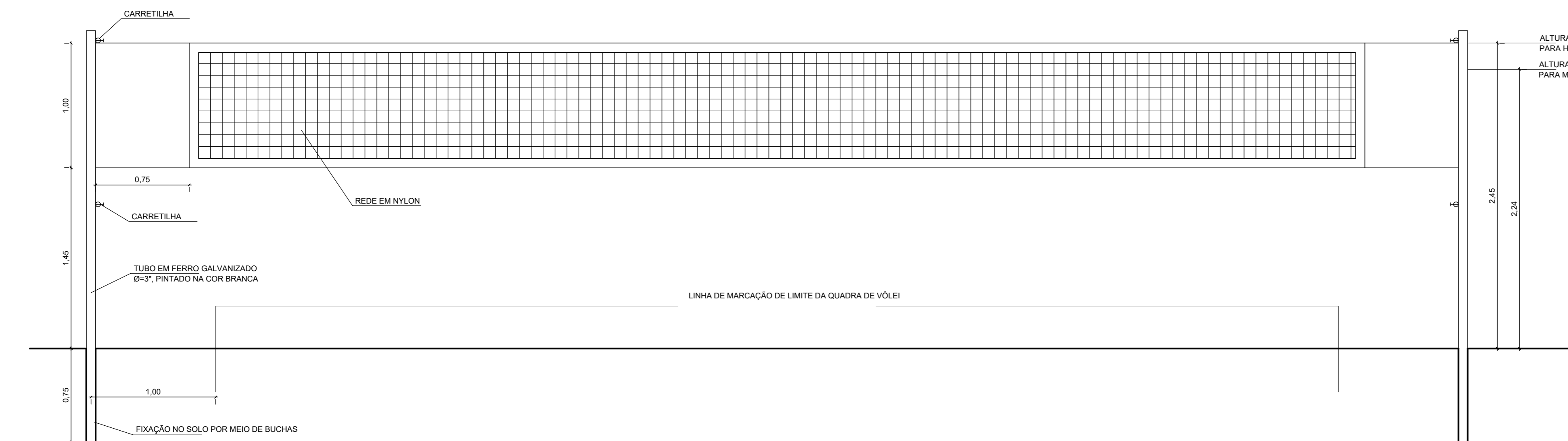
REDE DE VOLEIBAL ESCALA: 1/25
