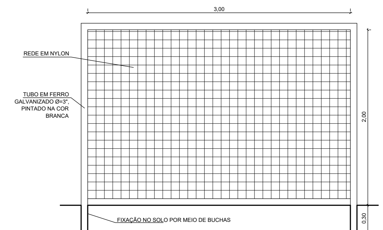
BALISA FUTEBOL - VISTA FRONTAL ESCALA: 1/25
