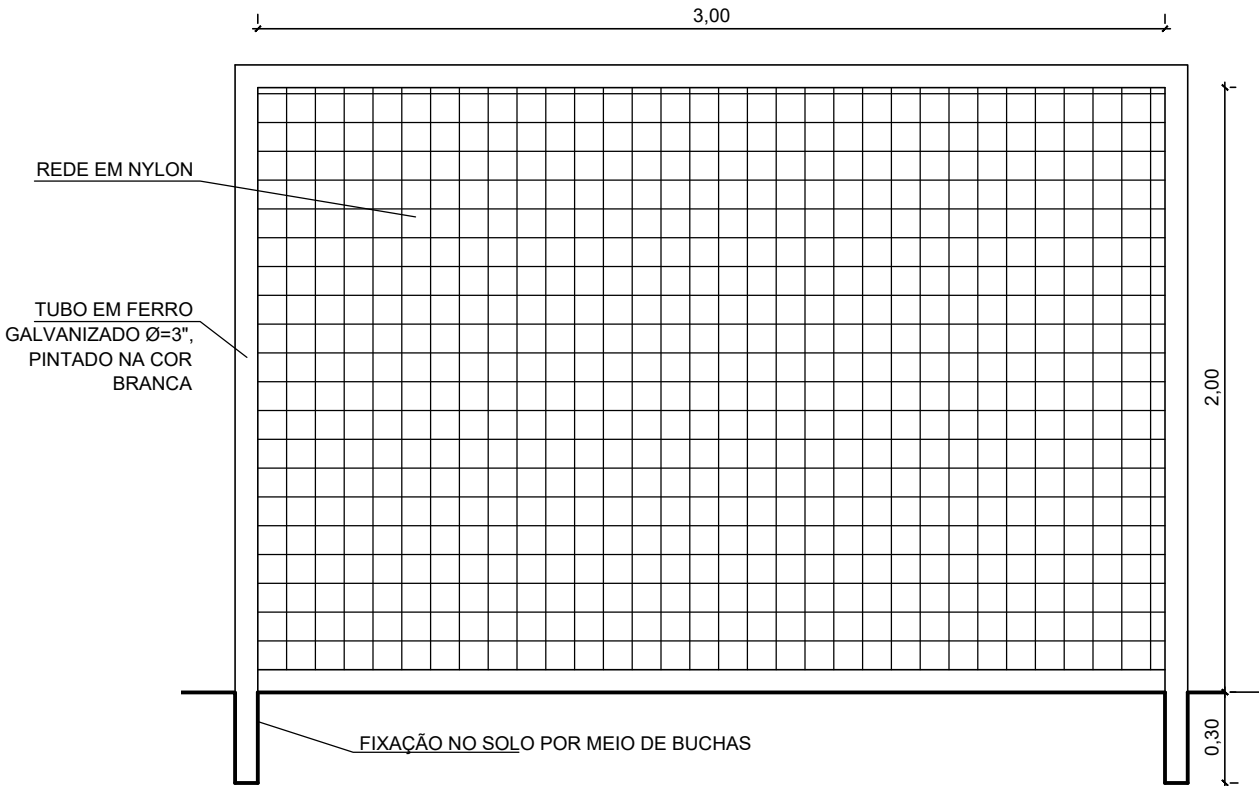
BALISA FUTEBOL - VISTA FRONTAL ESCALA: 1/25
