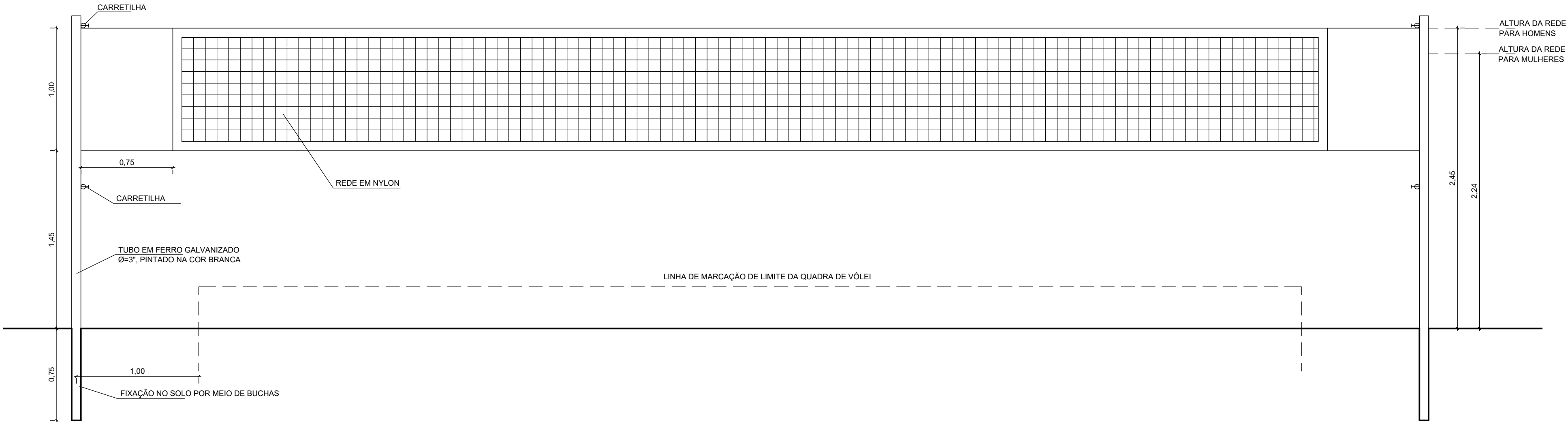
REDE DE VOLEIBAL ESCALA: 1/25
