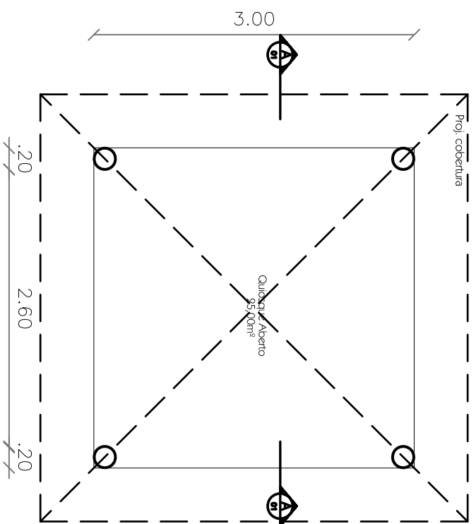
Planta Baixa
