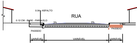
SEÇÕES TÍPICAS - RUAS DE CAPEAMENTO
