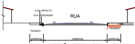
SECÇÃO TÍPICA RUAS RECAPEAMENTO
