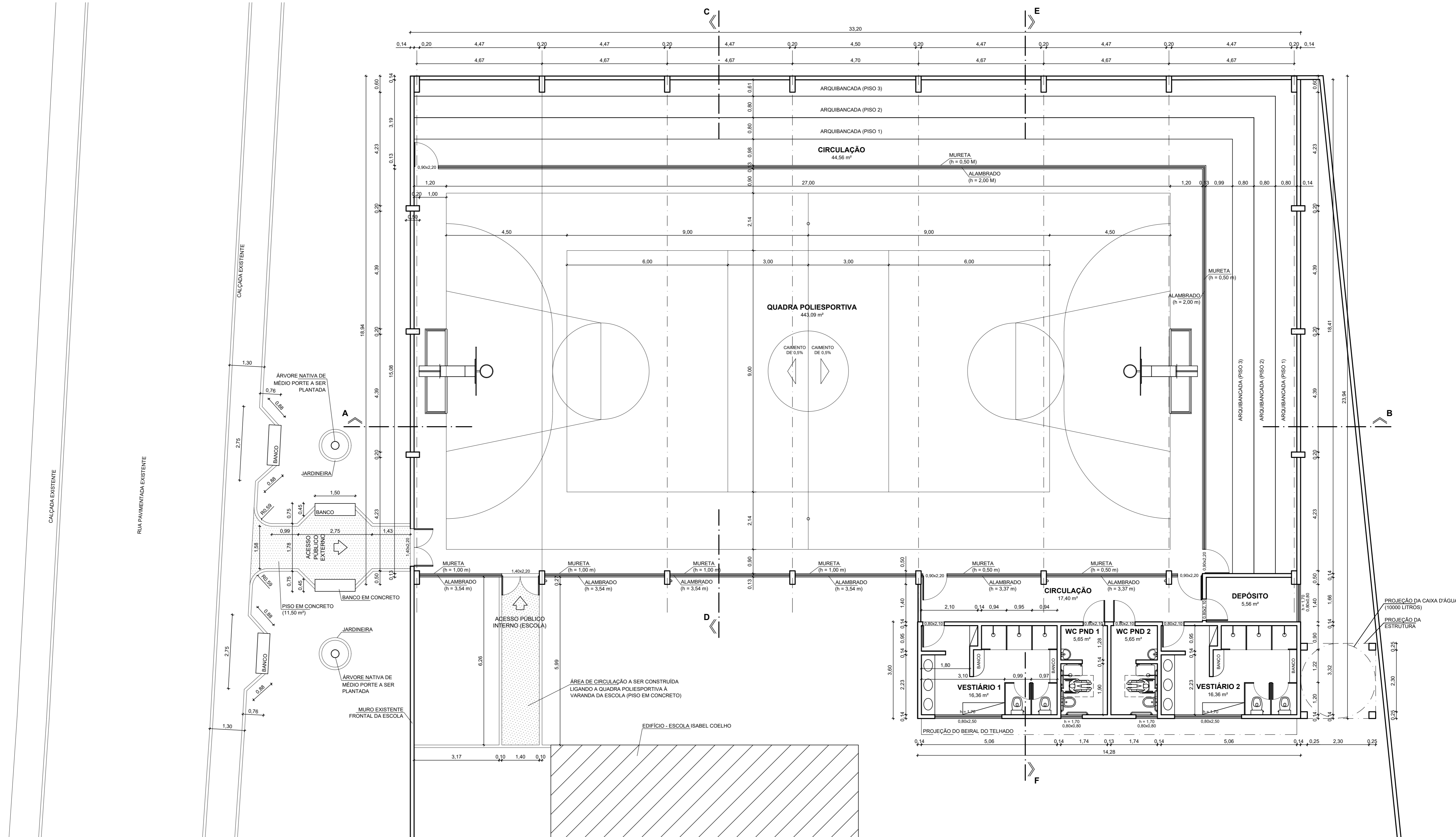
PLANTA BAIXA - QUADRA POLIESPORTIVA E VESTIÁRIO ESCALA: 1/100
