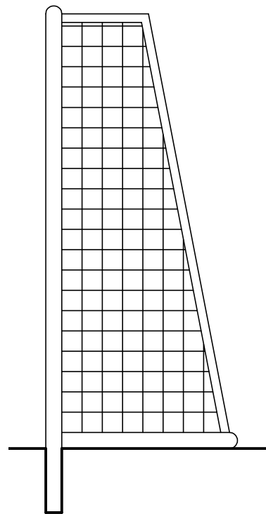
BALISA FUTEBOL - VISTA LATERAL ESCALA: 1/25
