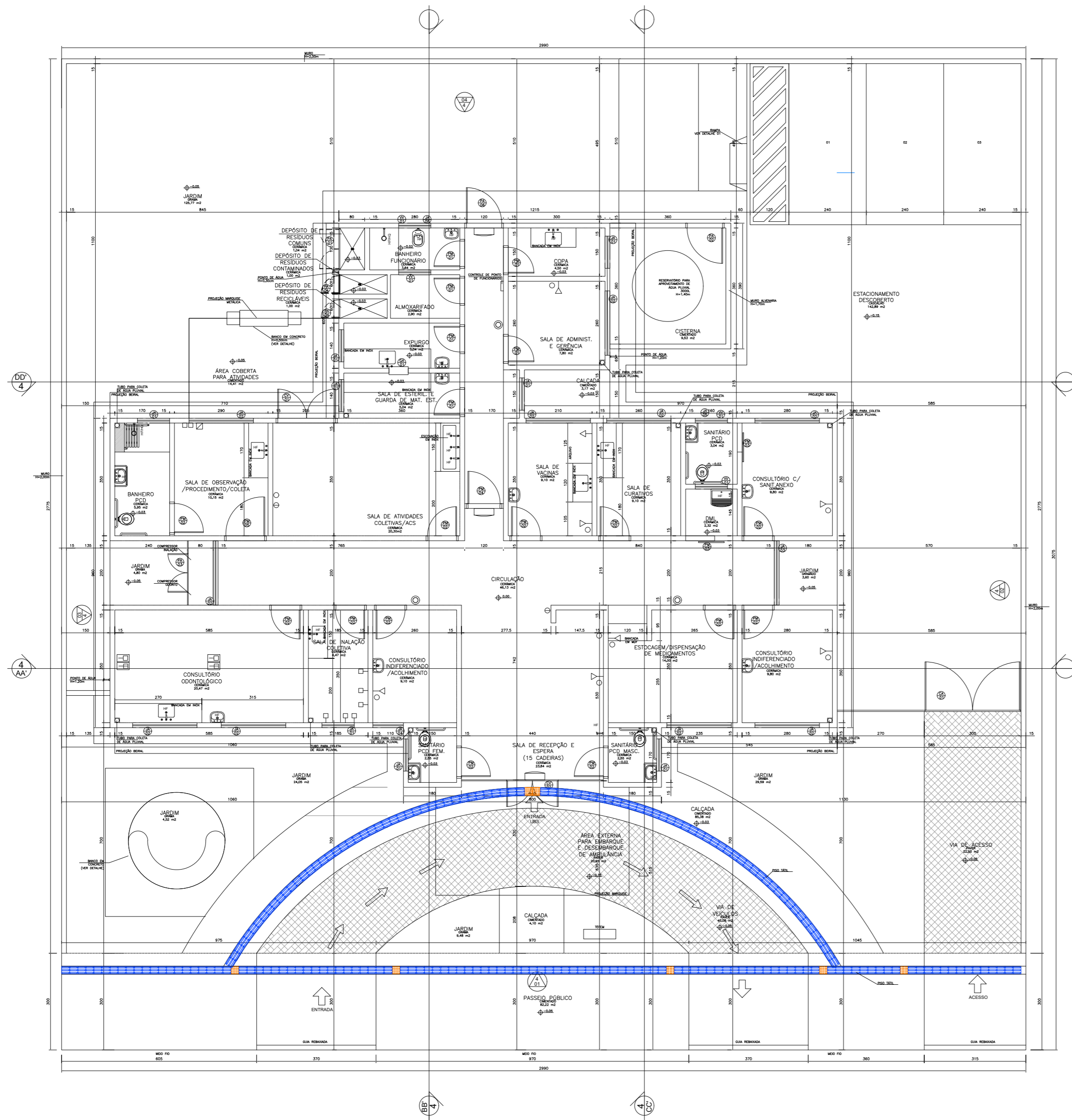
1 PLANTA BAIXA ESCALA 1/100
