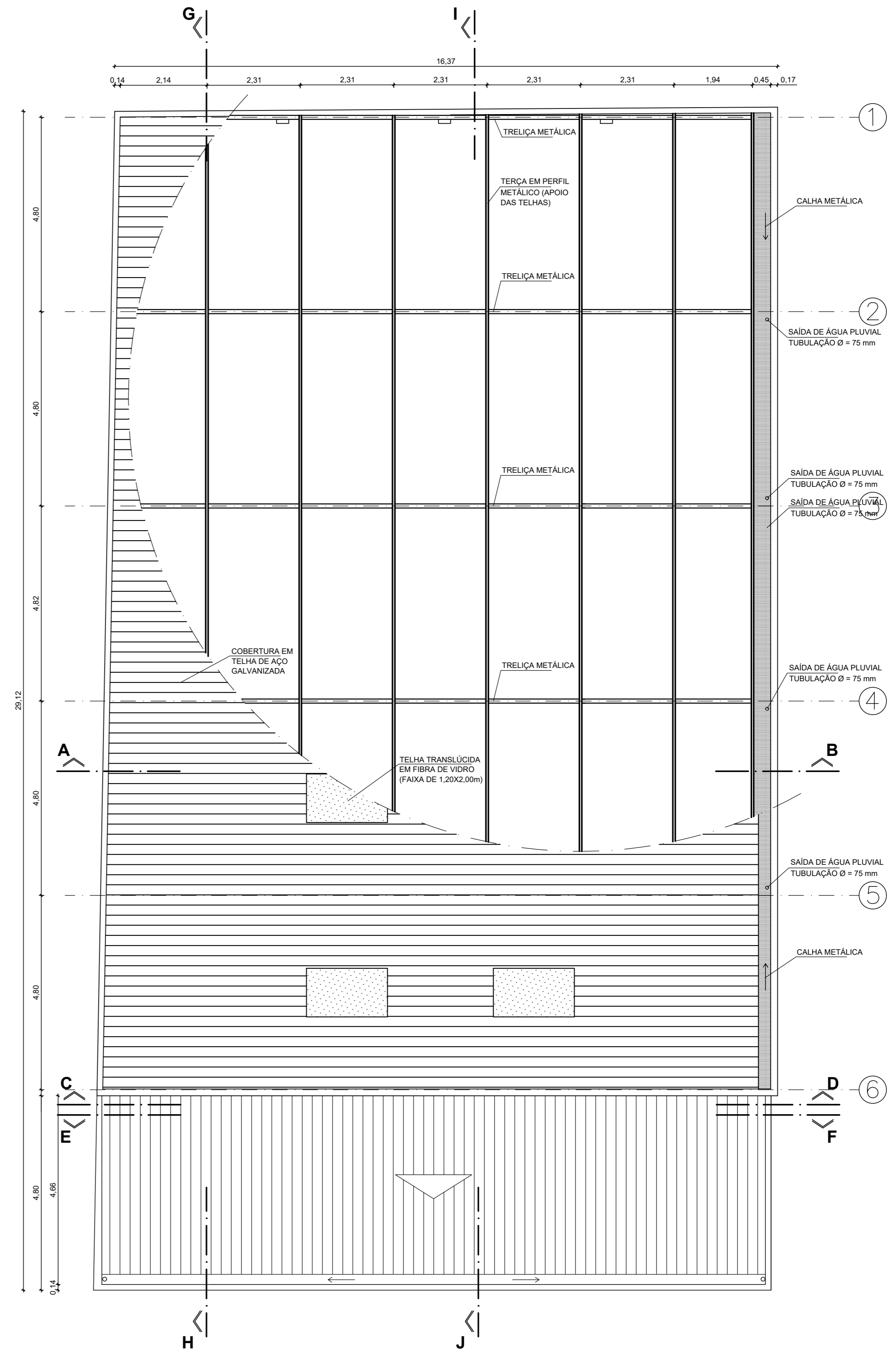
PLANTA DE COBERTURA - DETALHE ESCALA: 1/75
