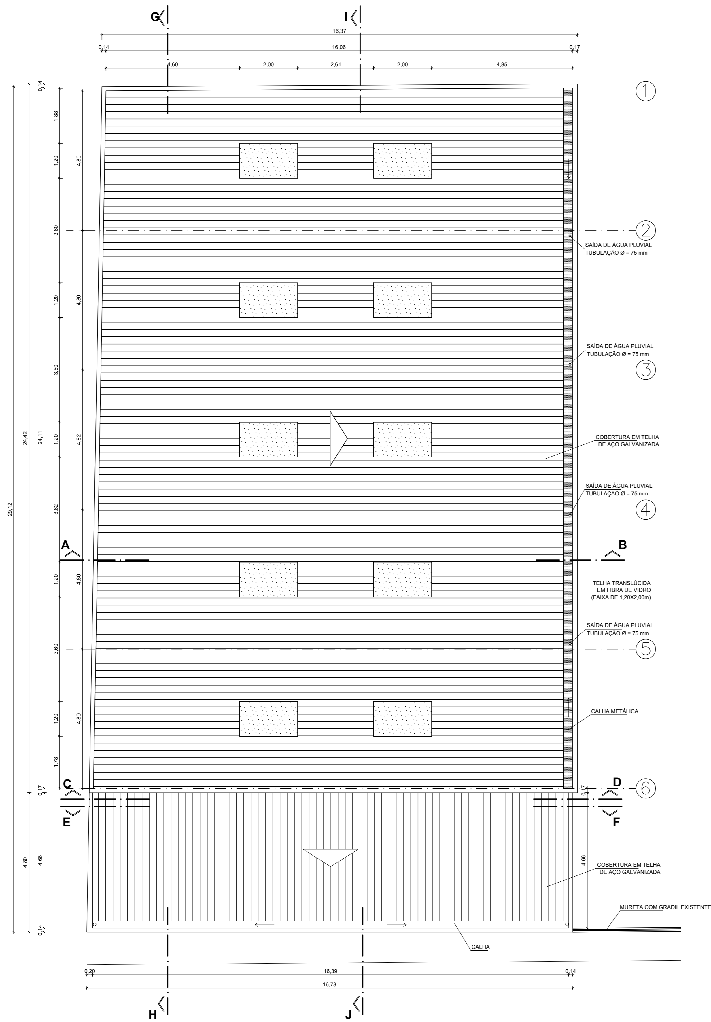
PLANTA DE COBERTURA ESCALA: 1/75
