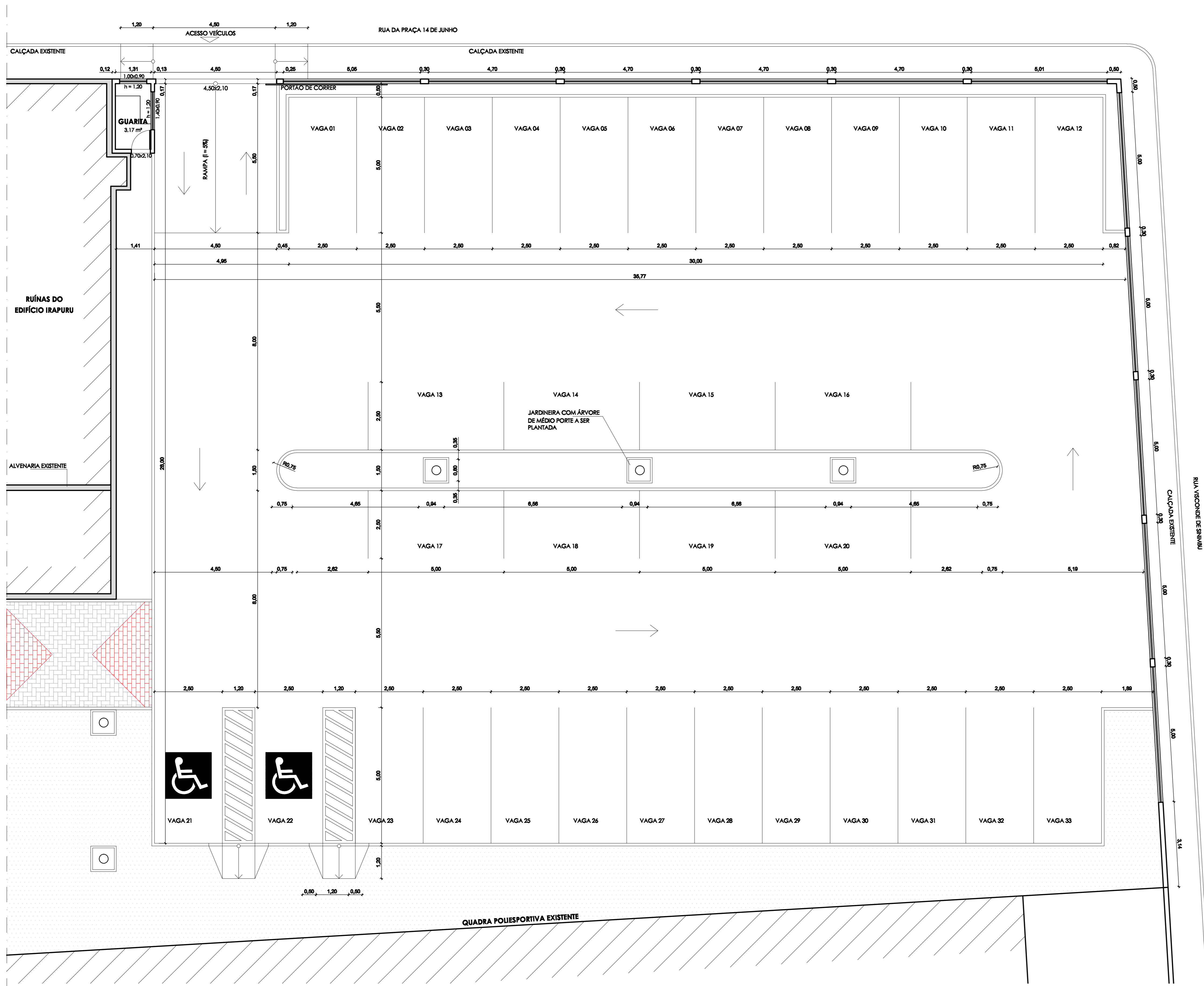
PLANTA BAIXA - ESTACIONAMENTO ESCALA 1/75
