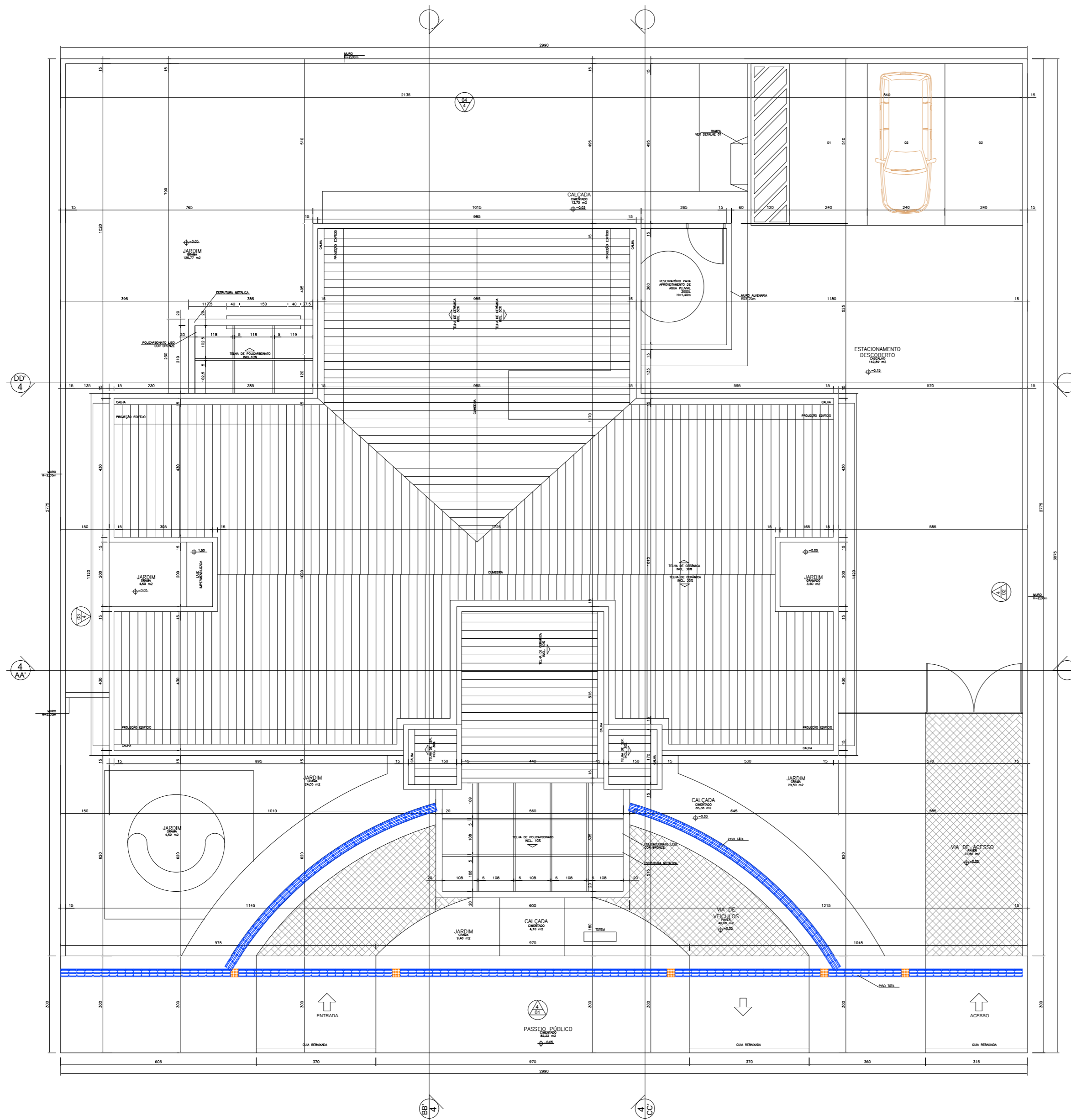
1 PLANTA DE COBERTURA ESCALA 1/100
