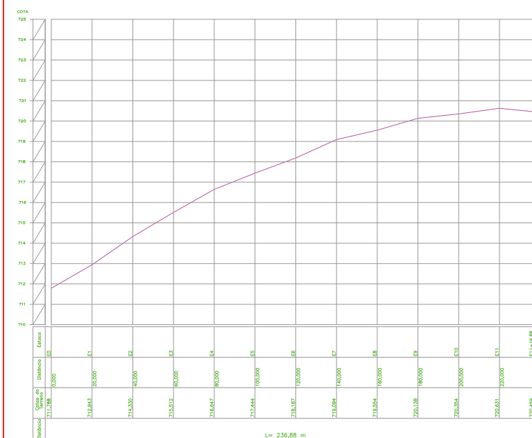
6 PERFIL LONGITUDINAL DO EIXO DA RUA ORÁCIO ALCÂNTARA DE ALMEIDA ESCALA 1/500
