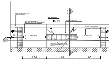
2 PLANTA BAIXA RAMPAS ACESSIBILIDADE
