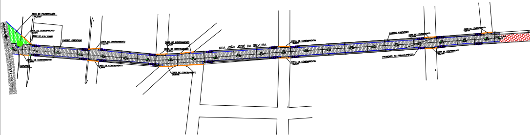
4 PLANTA DE PAVIMENTAÇÃO ESCALA: 1/750
