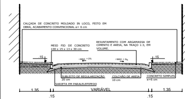
1 DETALHE DISCRIMINATIVO DA PISTA DE ROLAMENTO
