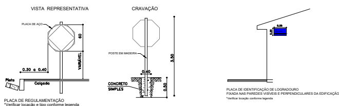
1 PLACAS DE SINALIZAÇÃO 1/5 ESCALA
