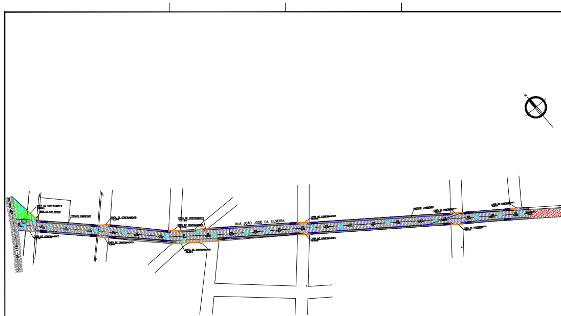
6 DRENAGEM SUPERFICIAL ESCALA: 1/750
