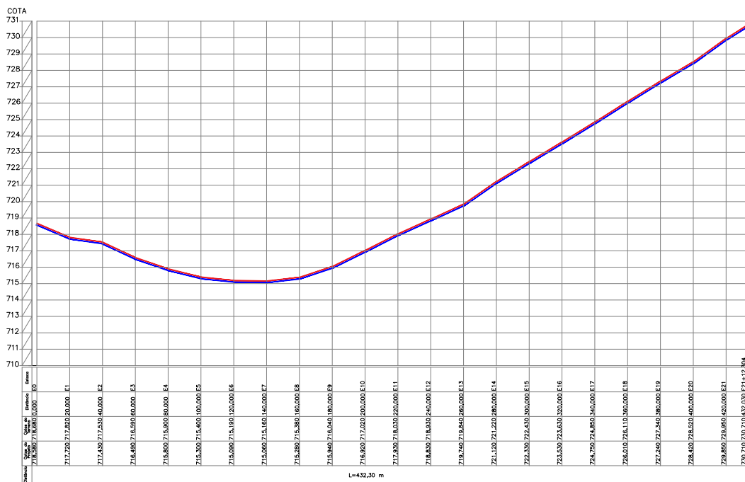
3 PERFIL LONGITUDINAL ESCALA: 1/750
