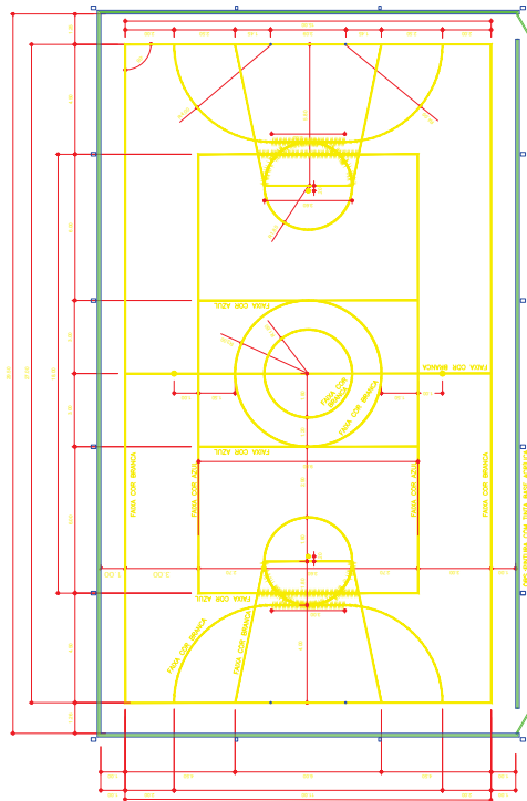
1 Demarcação do Piso ESCALA 1/100
