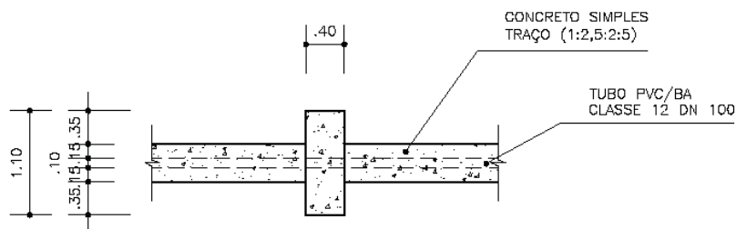
CORTE
