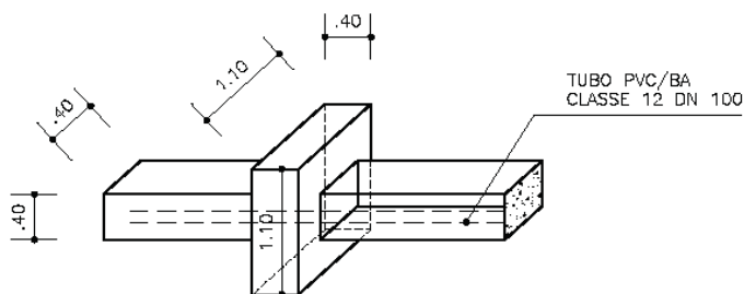
PERSPECTIVA
