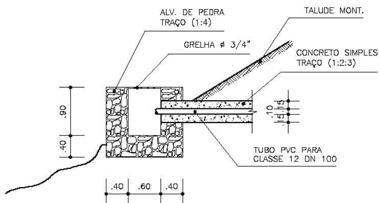
CORTE
